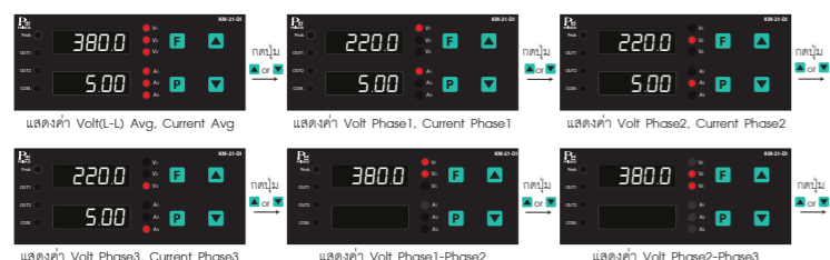
แสดงค่า Volt(L-L) Avg, Current Avg
